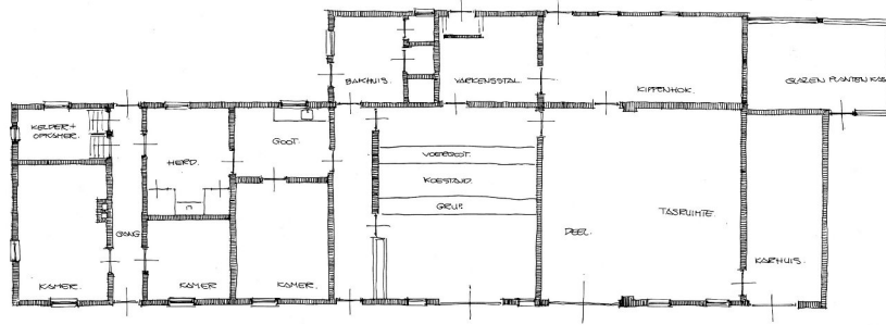
PLAAT GROND
