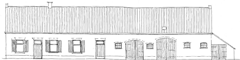
NOORD GEVEL
