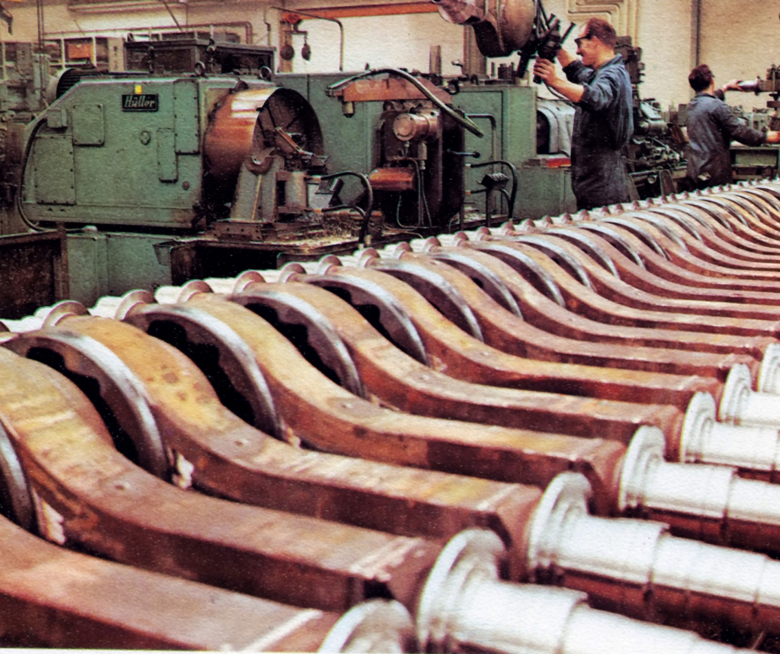
achterassen en plaatsen differentieel
